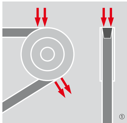
Frecarea pe flancuri la intrare și ieșire, pierderi de frecțiune interioară datorită fenomenului de histerezis.
